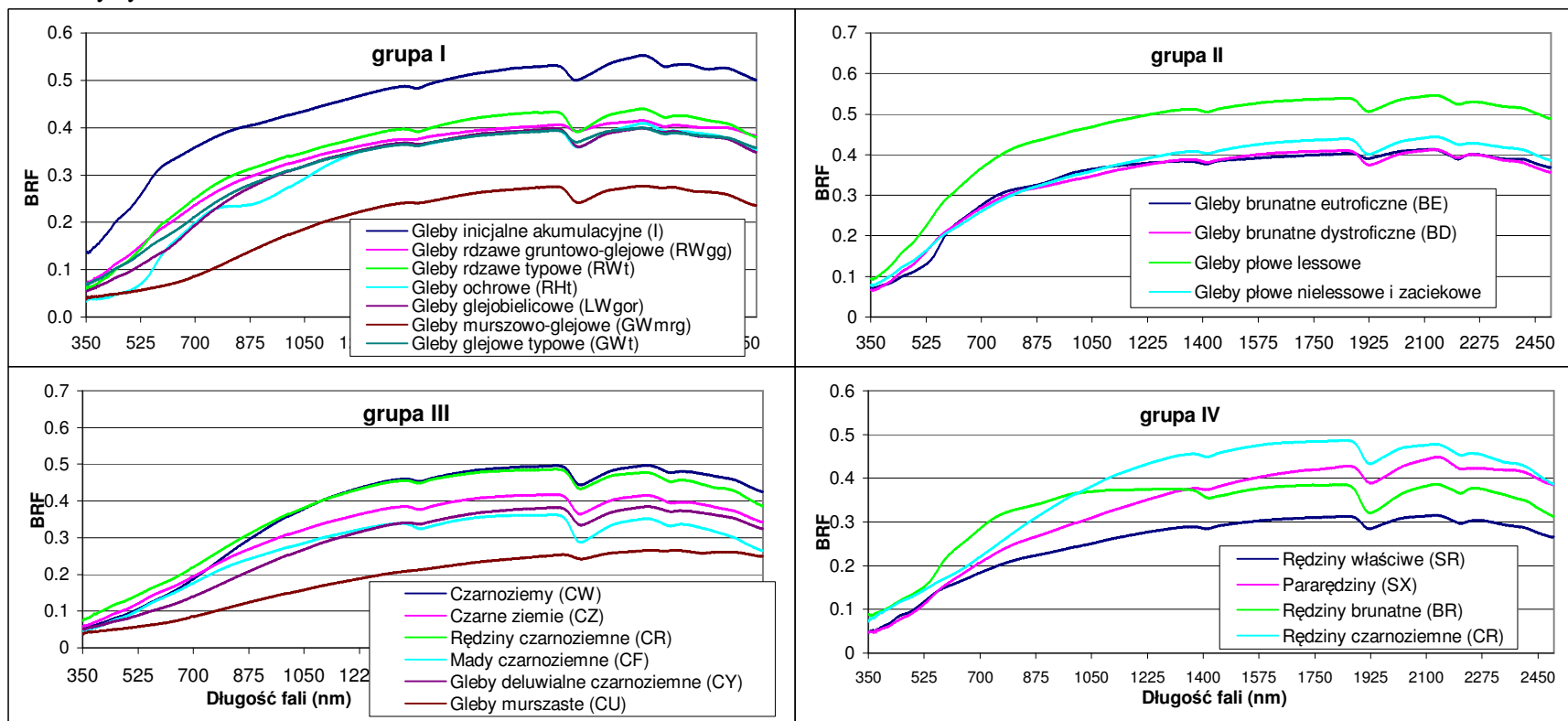
Ryc. 4. Krzywe spektralne gleb z siedmiu rzędów taksonomicznych uzyskane w pomiarach DRS pogrupowane według rodzajów materiałów macierzystych.
