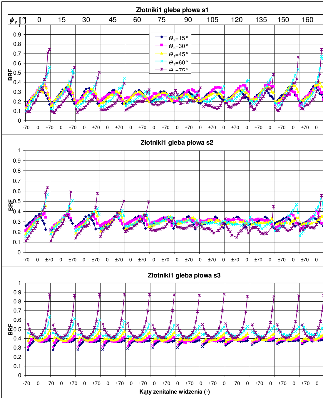
Ryc. 9. Wartości wskaźników BRF trzech powierzchni glebowych o trzech różnych poziomach szorstkości s1, s2 i s3 dla fali o długości 850 nm w funkcji kąta zenitalnego widzenia \theta_v w dwunastu pionowych płaszczyznach obserwacji ( \phi_v ) przy pięciu położeniach zenitalnych lampy ( \theta_s ), zarejestrowane w trakcie laboratoryjnych pomiarów goniometrycznych.
